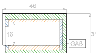
Sezione trasversale
